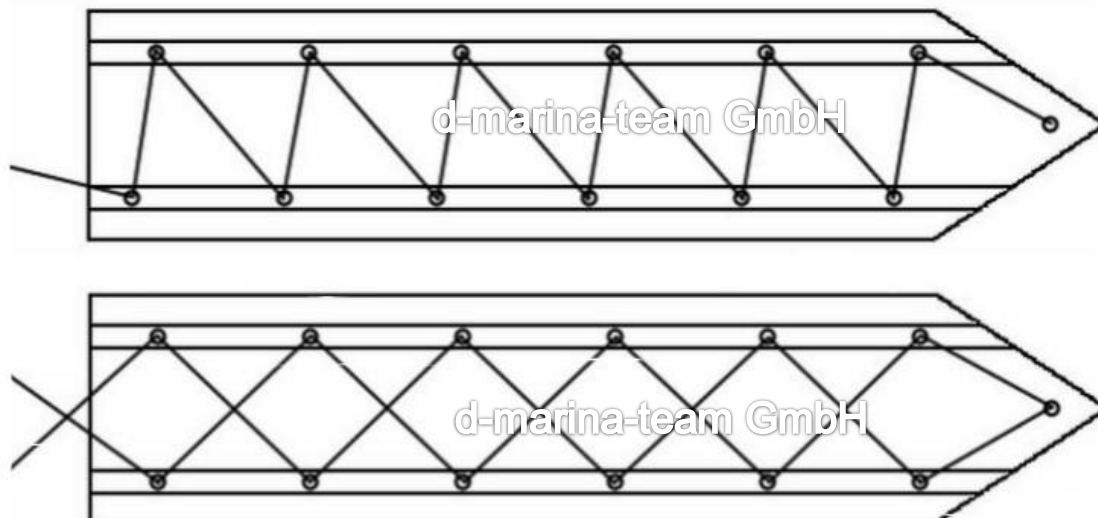
Beispiel einer Schnürung für Rollfockpersennig
