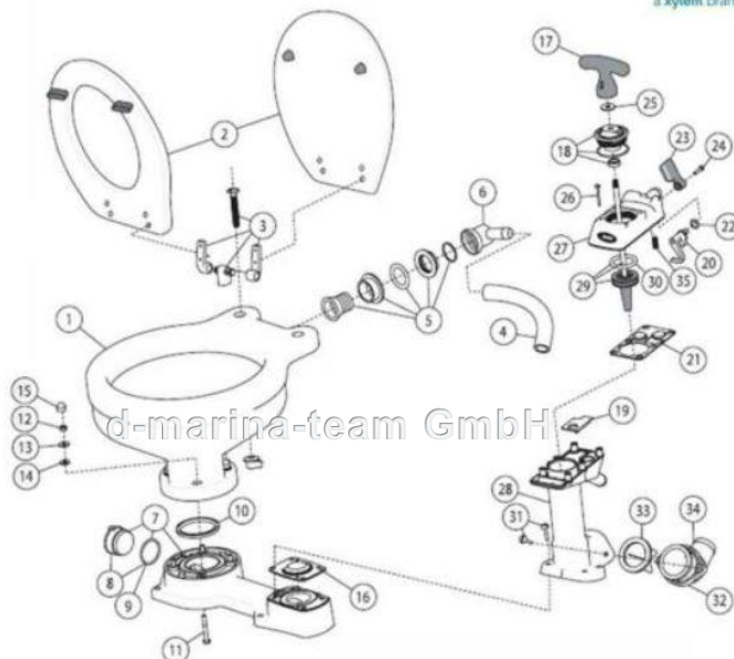
Baureihe / Series 29090 & 29120
