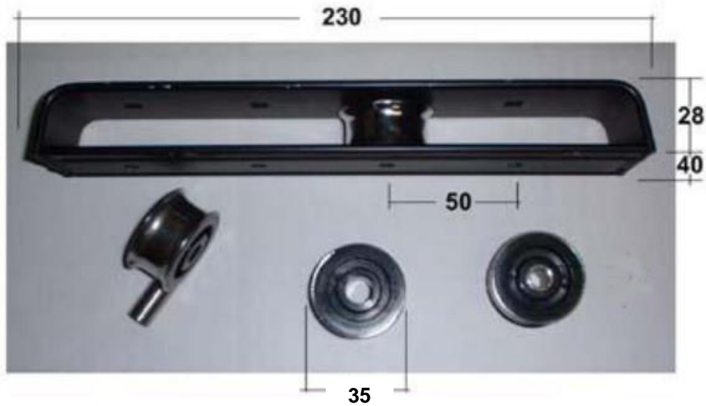
Aluminiumgehäuse schwarz
